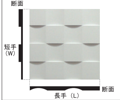
市松の断面形状
