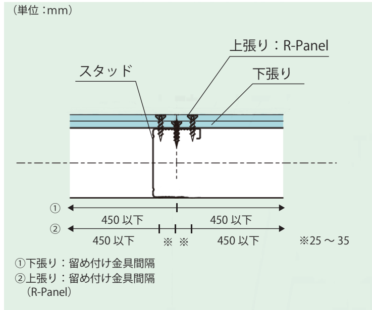
内壁：水平方向断面
